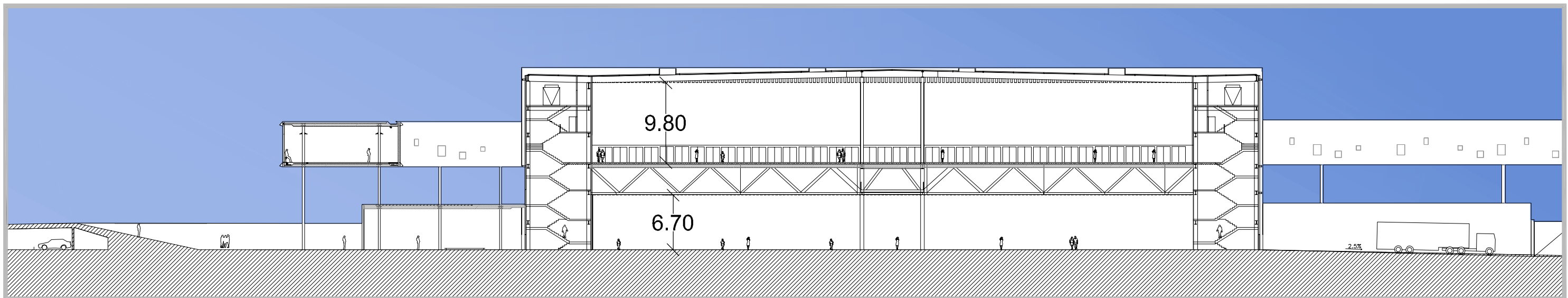
SECTION B-B' / SECCIÓN B-B'
